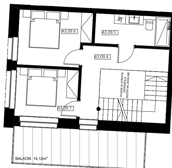
PIĘTRO
